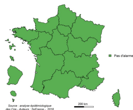
Figure 2 : Niveau d'alerte régional en semaine 47/2018
